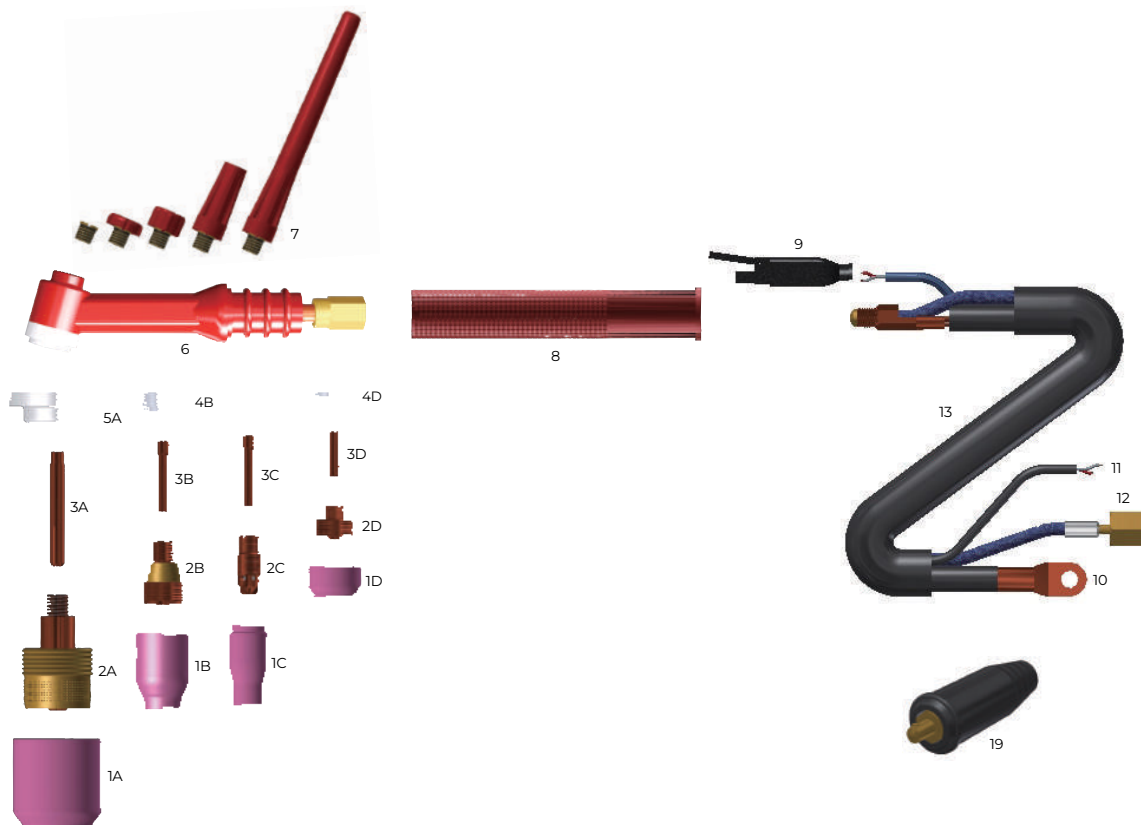
WT9 风冷两件式零件/
