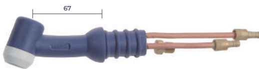
WON350A 水冷柔性焊枪WT26FW 6-80-7
