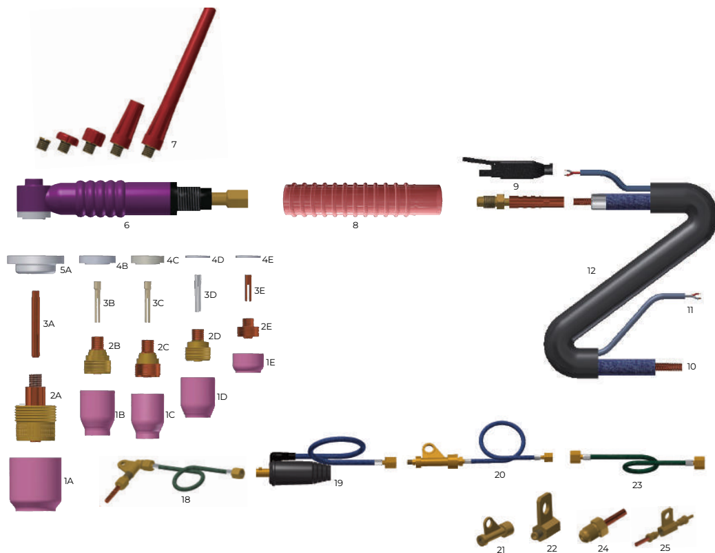
WT80A&amp;125A&amp;150A&amp;170A 风冷一体式锅炉零件清单
