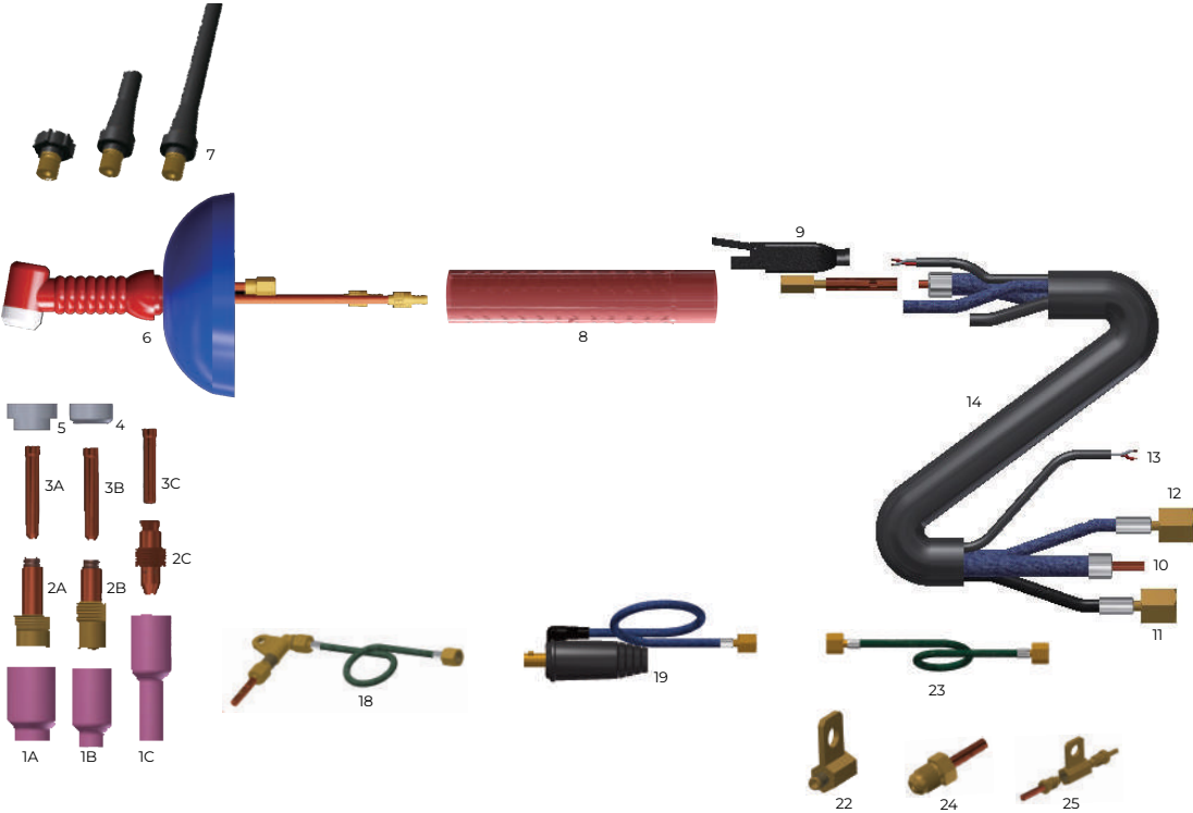
WT40&400A 大容量水冷配件清单
