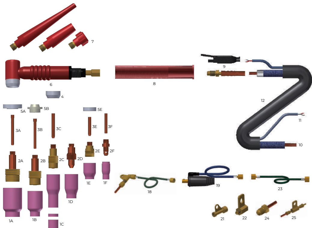
WT17 风冷一体式零件/
