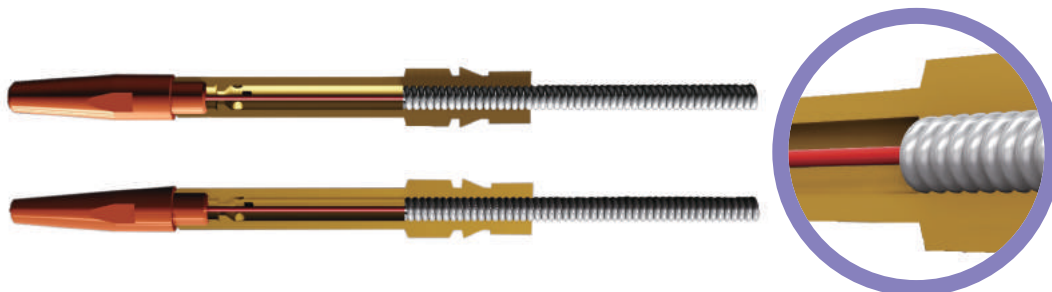
用于防止实心线短路的气体分流器
