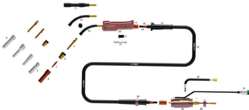
Các biến thể có sẵn
