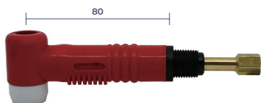
WON 170A Mỏ hàn cổ mềm làm mát bằng không khí WT-170F
