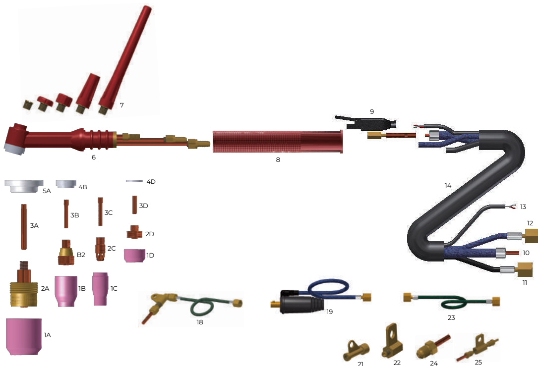
WT20&amp;180A Danh mục phụ tùng làm mát bằng nước
