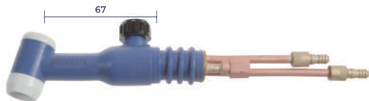
WON350A Mỏ hàn có van, làm mát bằng nước WT18VW 6-78-1
