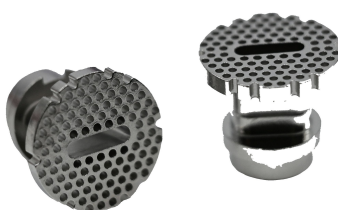
Tấm lọc chống bắn tóe
