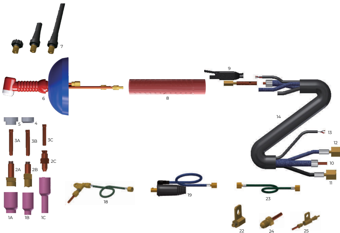
WT40&400A Danh mục phụ tùng công suất lớn, làm mát bằng nước
