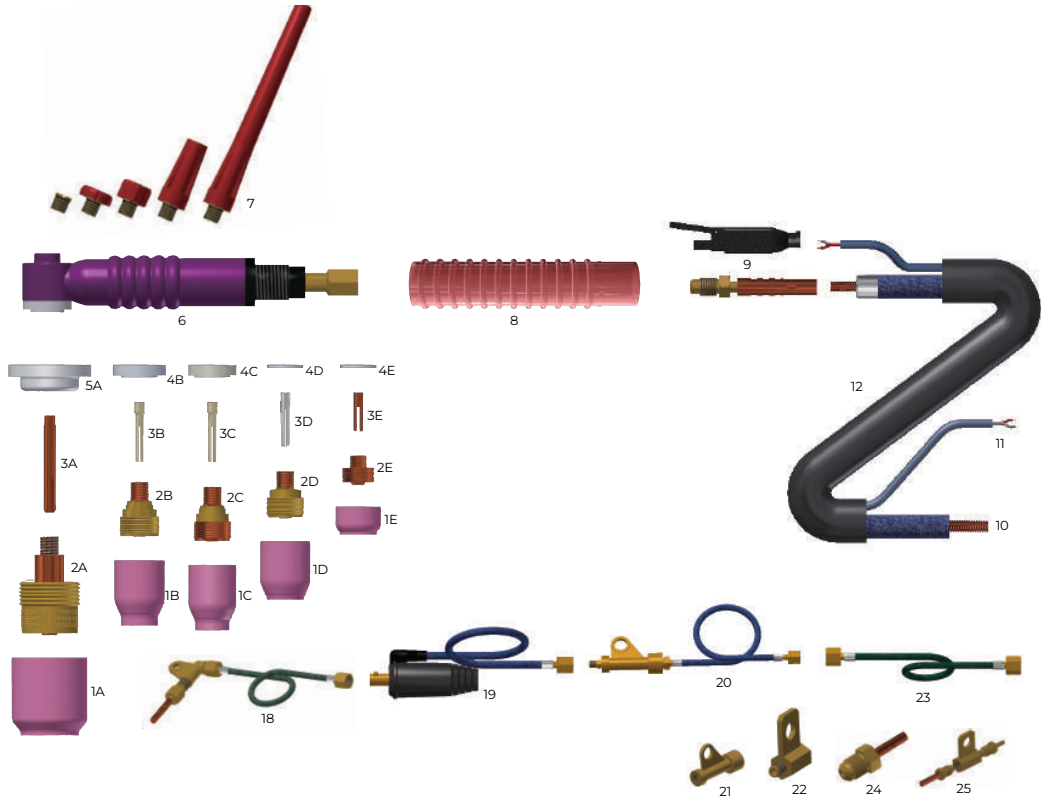
WT80A&125A&150A&170A Air-cooled One-piece Boiler Parts / WT80A&125A&150A&170A 원피스 보일러용 부품 명칭
