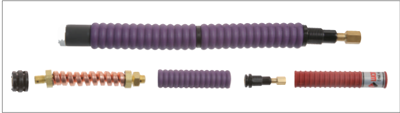
WON180A Air-cooled Flexible Components WON180A 공냉 후렉시블 구성 요소
