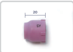
Large Mini Gas Lens Body Ceramic WTS261805 대구경 미니 가스렌지 바디 세라믹 WTS261805
