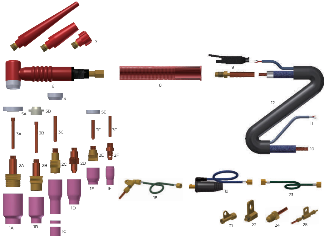
WT17 Air-cooled One-piece Parts / WT17 원피스 공냉 부품 명칭
