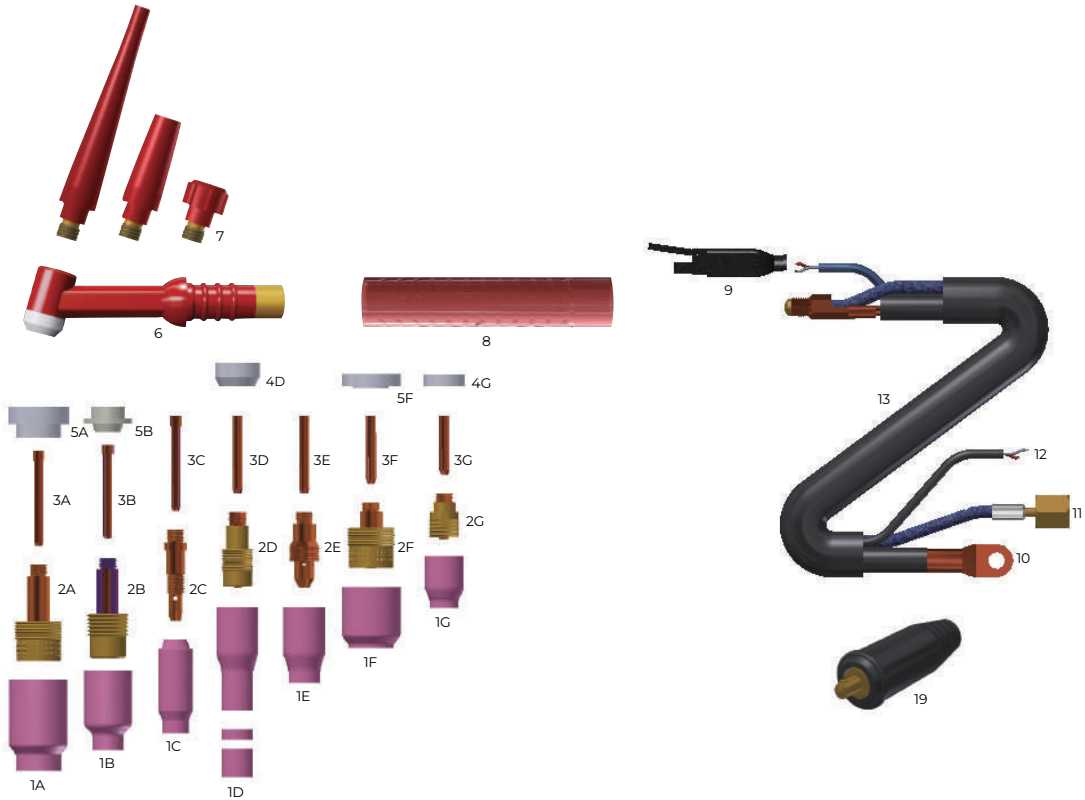
WT26&200A Air-cooled Two-piece Parts / WT26&200A 투피스 공냉 부품 명칭
