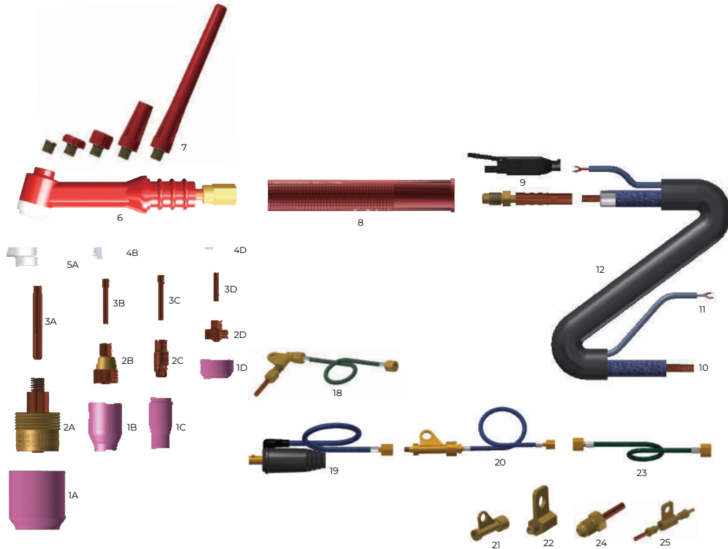
WT9 Air-cooled One-piece parts / WT9 공냉원피스 부품 명칭
