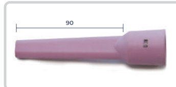
Narrow Gap Gas Lens Body Ceramic Nozzle 90mm WTS261807 내로갭 가스렌지 바디 세라믹 노즐 90mm WTS261807
