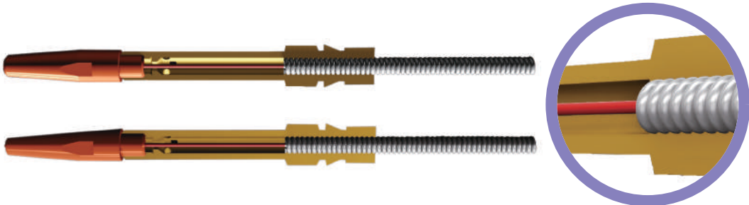
Solid Wire Short Preventing Diffuser 솔리드 와이어 쇼트 방지용 디퓨샤
