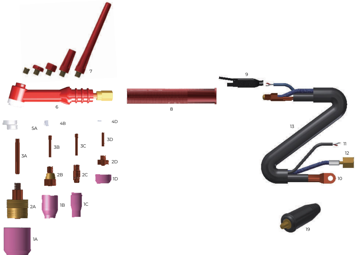
WT9 Air-cooled Two-piece Parts / WT9 공냉토티스 부품 명칭
